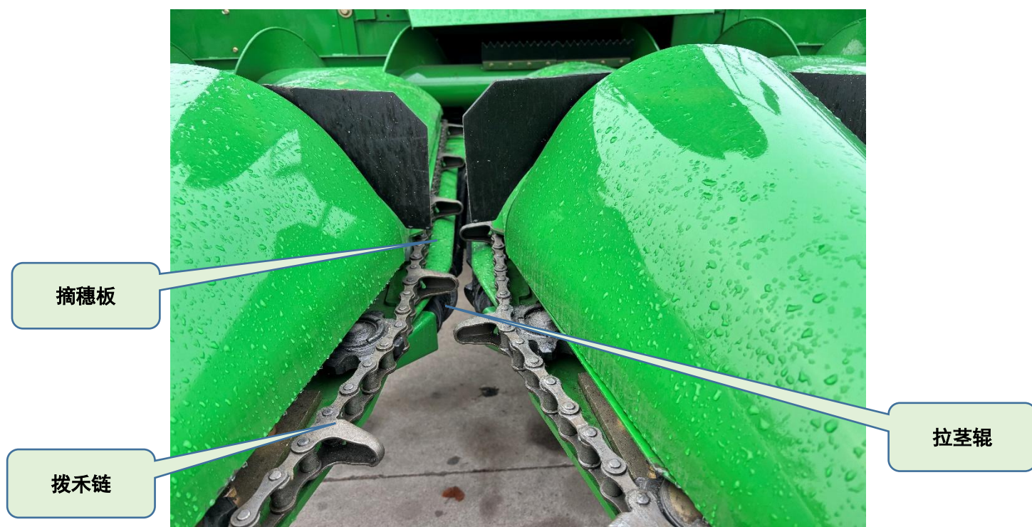
6、摘穗机构（摘穗板式）
