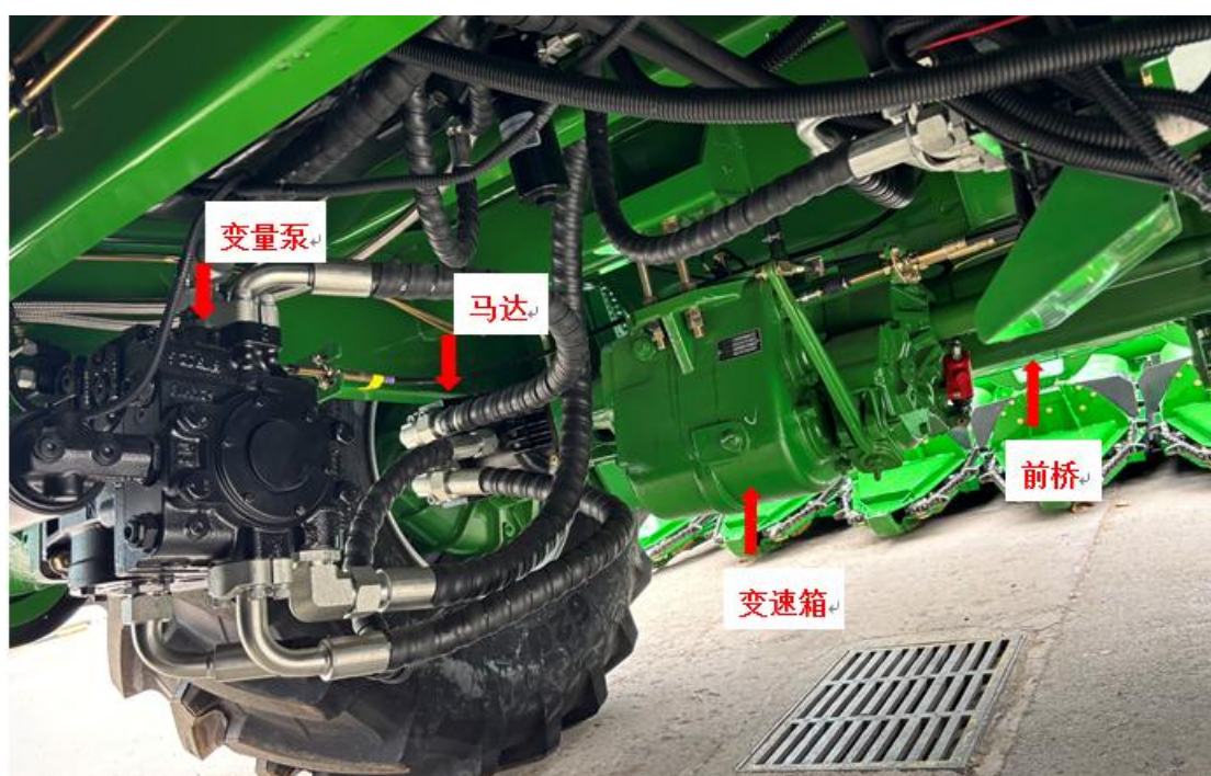
8、驱动方式（前轮：液压驱动）
